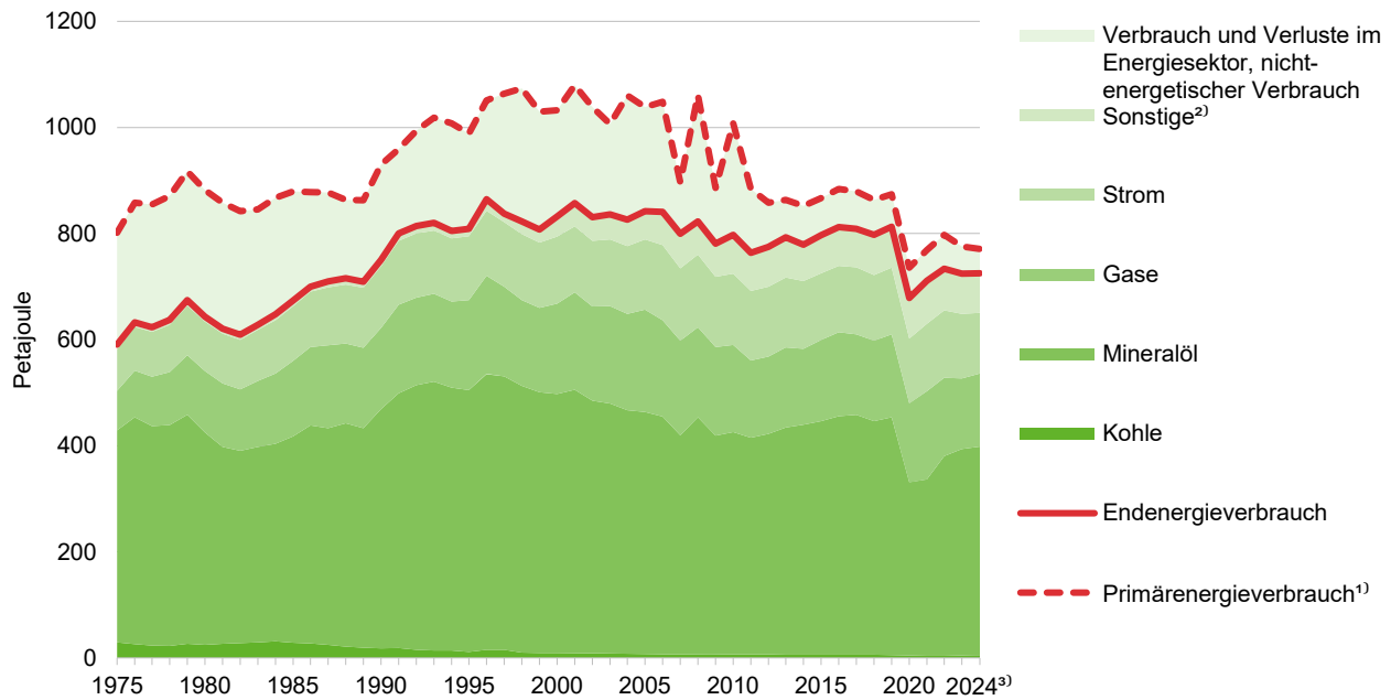
Abb. 1: Primärenergieverbrauch in Hessen 1975 bis 2024 nach Energieträgern
