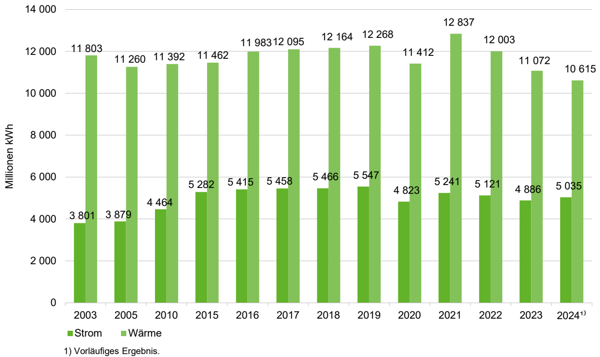
Abb. 3: Strom- und Wärmeerzeugung aus Kraft-Wärme-Kopplung in Hessen 2003 bis 2024 (Kraftwerke der allgemeinen Versorgung und Industriekraftwerke)
