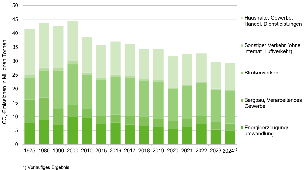
Abb. 4: Entwicklung der energiebedingten CO 2 -Emissionen in Hessen 1975 bis 2024 nach Verbrauchssektoren
