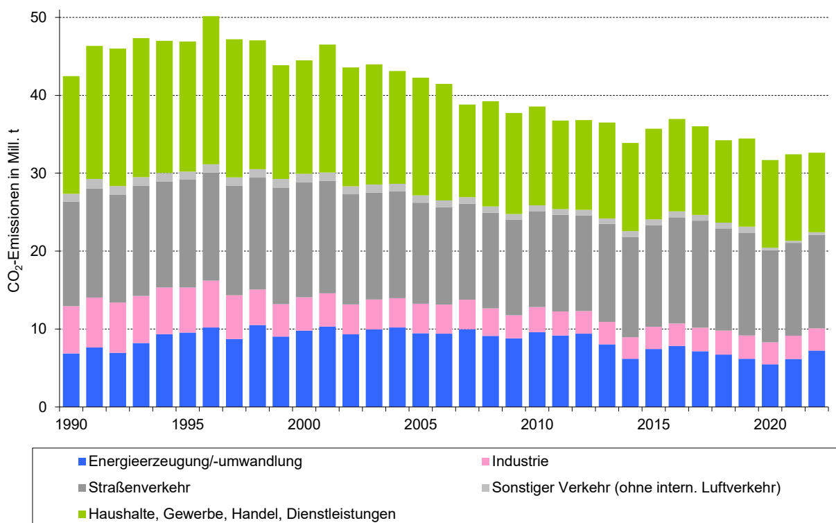
Abbildung 2 Energiebedingte CO 2 -Emissionen in Hessen von 1990 bis 2022 nach Sektoren
