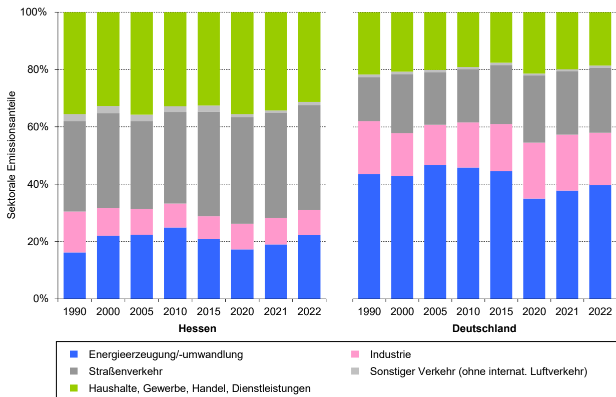
Abbildung 3 Sektorale Struktur der energiebedingten CO 2 -Emissionen in Hessen und Deutschland von 1990 bis 2022
