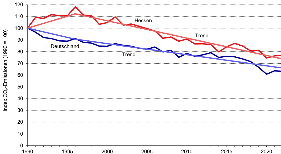
Abbildung 1 Energiebedingte CO 2 -Emissionen in Hessen und Deutschland von 1990 bis 2022
